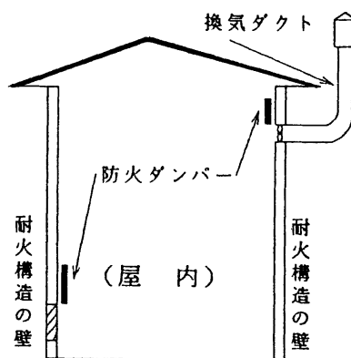
第17-4図 防火ダンパーの設置例
