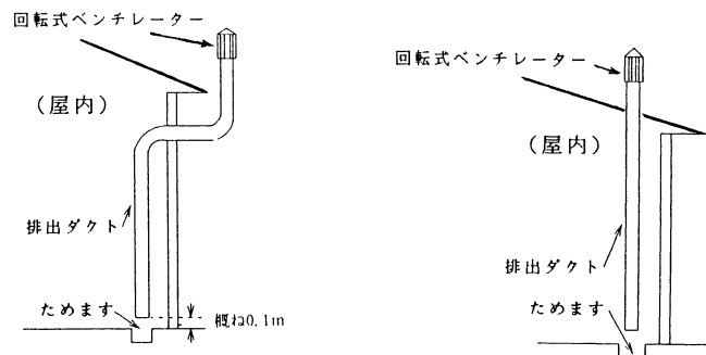
第17-6図 強制排出設備の例
