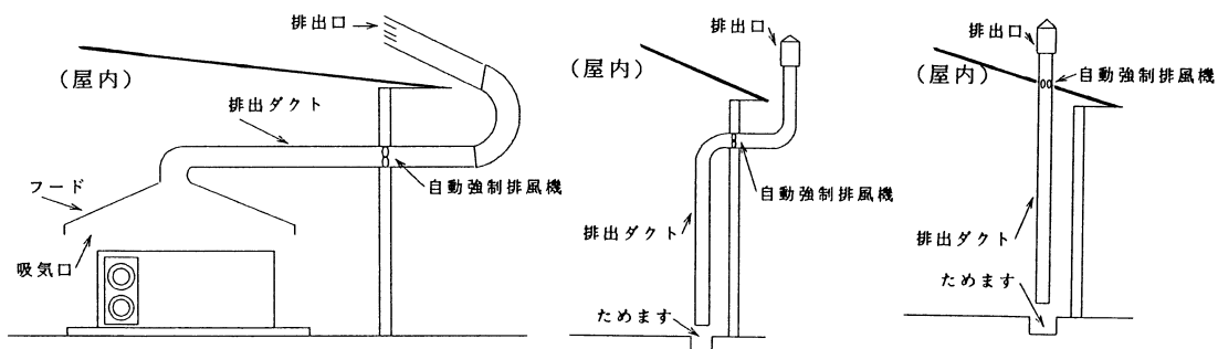
第17-5図 自動強制排出設備の例
