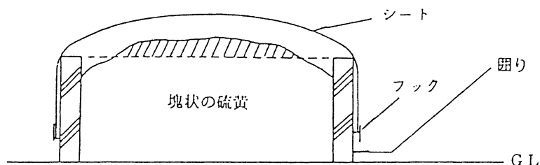
第12-4図（不可の例）
