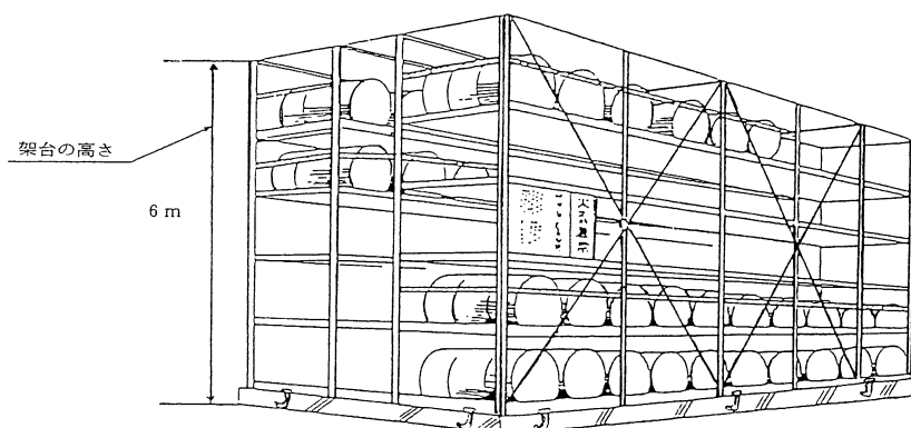
第12-2図 架台の高さ
