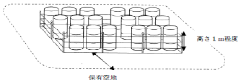
第12-1図 さくを設けた場合の例
