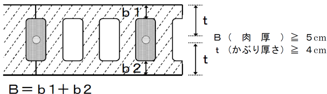
第6-1図 コンクリートブロック造の例
