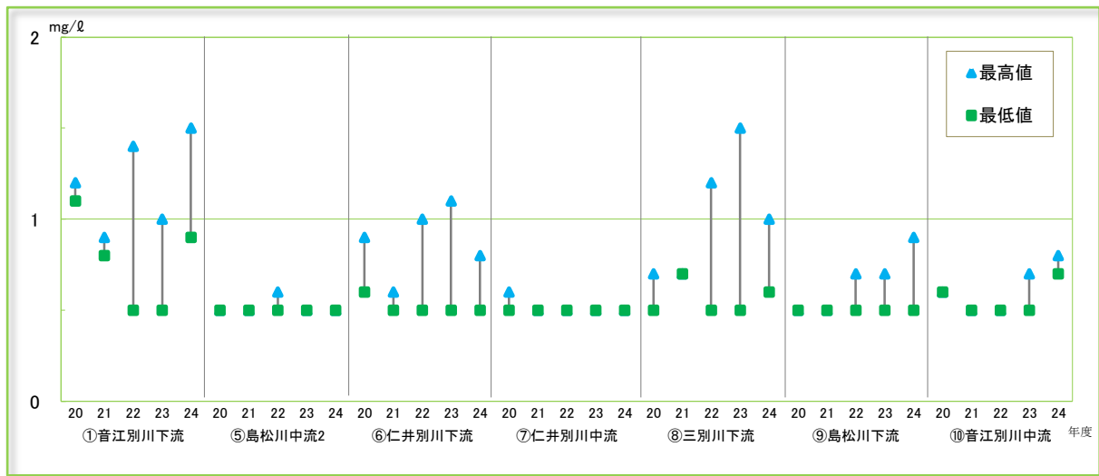
図 3-6 島松川水系における BOD 値の経年変化
