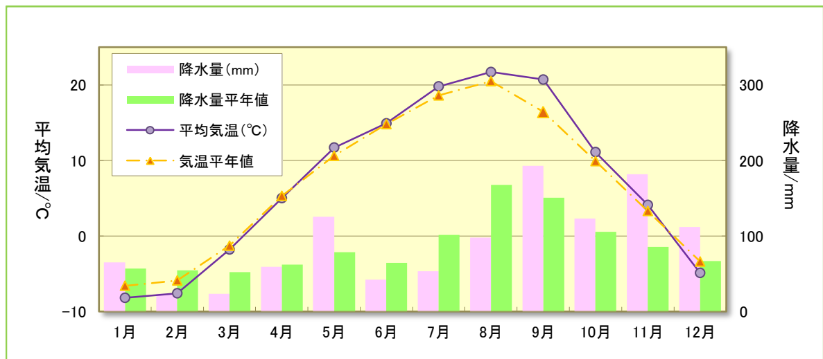
図 1-3 平成 24 年の平均気温と降水量
