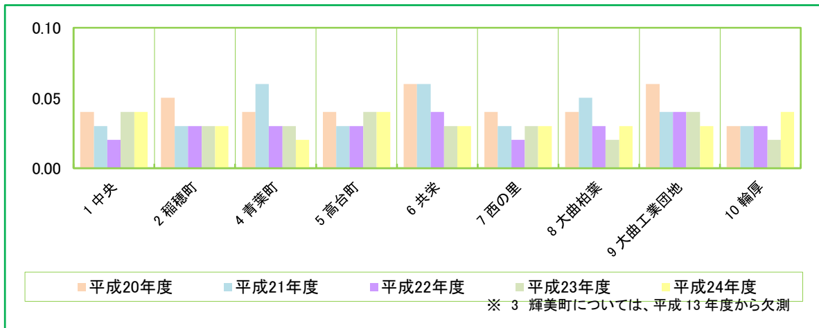
図3-1 二酸化鉛法によるいおう酸化物の測定結果(単位:SO 3 mg/100cm 2 /日)
