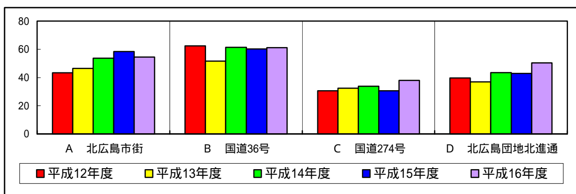
図 3 - 2 窒素酸化物の測定結果（単位：NO 2 μg/100cm 2 /日、測定結果の詳細：表 3 - 4 参照）
