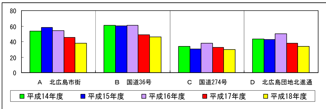
図 3-2 窒素酸化物の測定結果 (単位: NO 2 μg/100cm 2 /日、測定結果の詳細: 表 3-4②参照)
